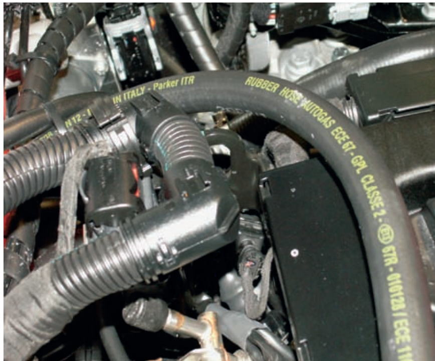
Sauber und knickfrei verlegt – bei WOW-Schulungen wird besonders auf den korrekten Einbau der Gasanlage geachtet
